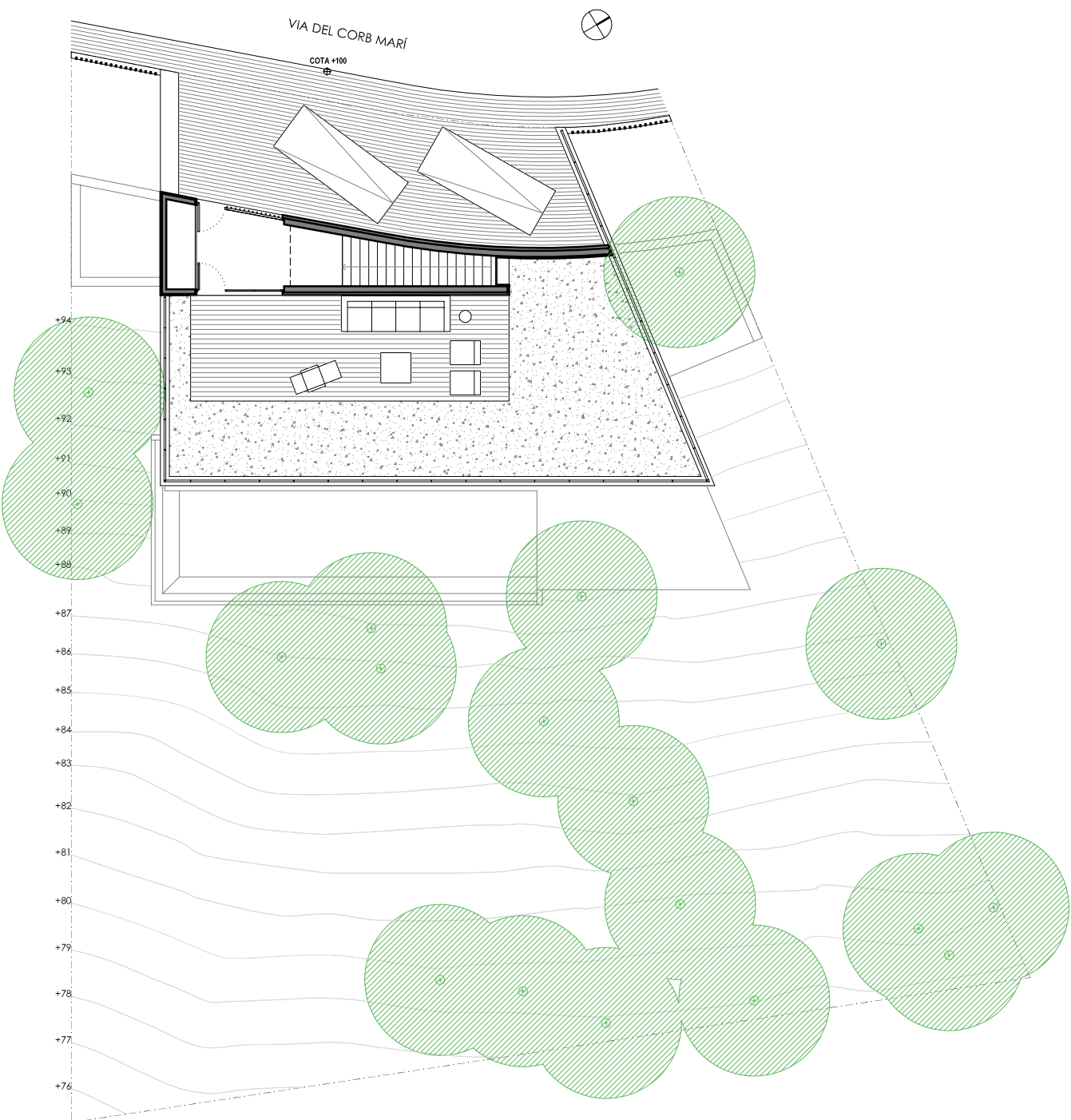
PLANTA COBERTA (ACCÉS) - E 1:200
