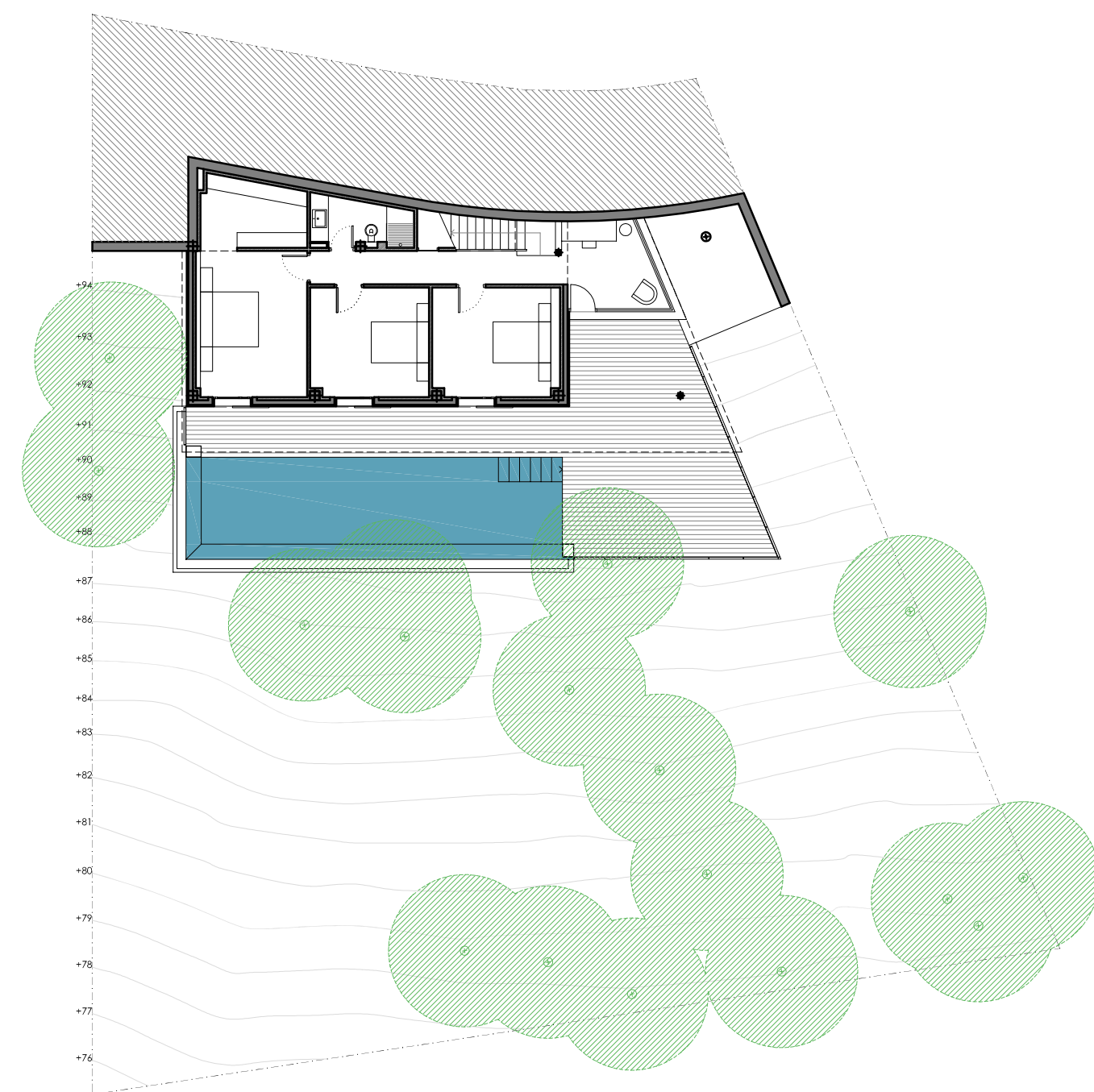
PLANTA BAIXA - E 1:200
